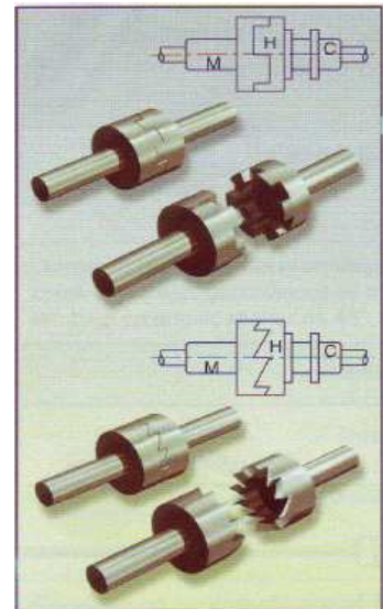
Fig. 4. Distintos modelos de embrague de dientes.
