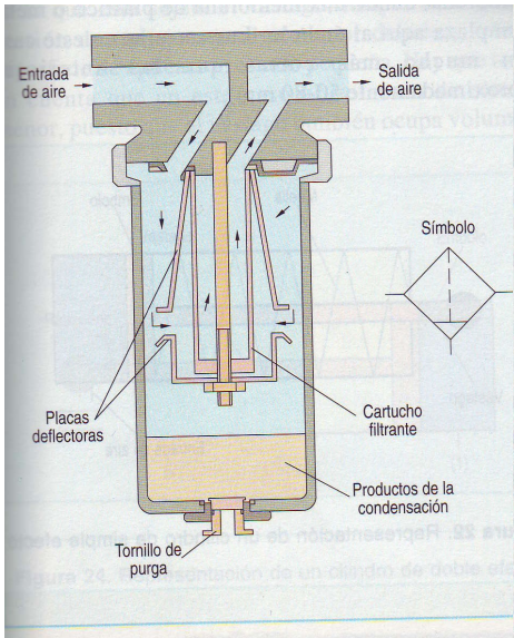
Figura 19. Estructura y símbolo del filtro
